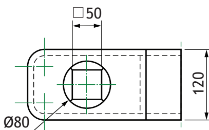
END ELEVATION
