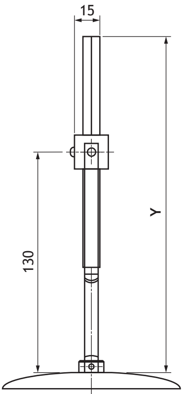
END ELEVATION
